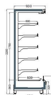
PEARL 2200 / 950 / 325
