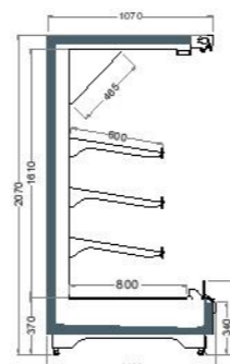
PEARL 2070 / 1100 / 340
