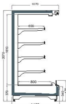
PEARL 2070 / 1100 / 340
