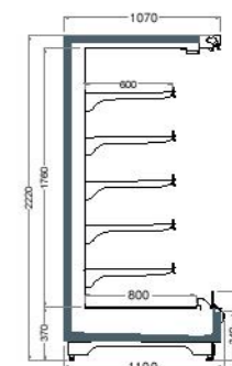
PEARL 2220 / 1100 / 340
